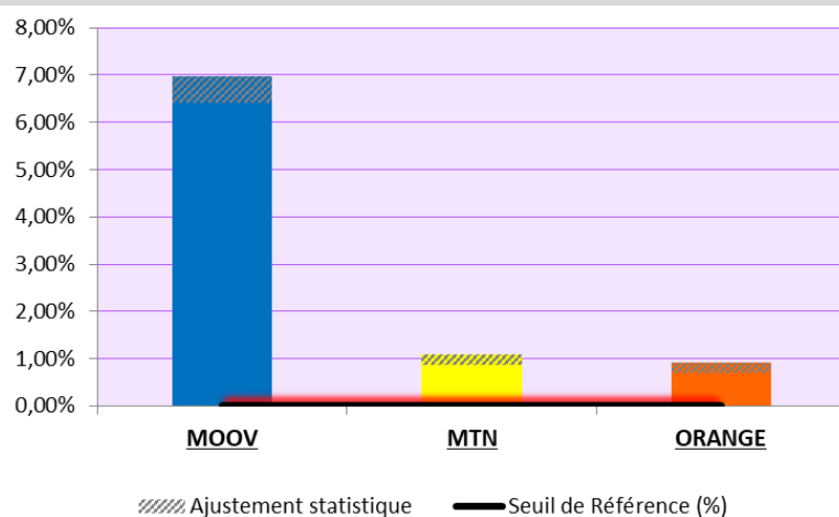
Taux de débit moyen en Downlink par session d'utilisateur inférieur à 512 kb/s (Tddd)
