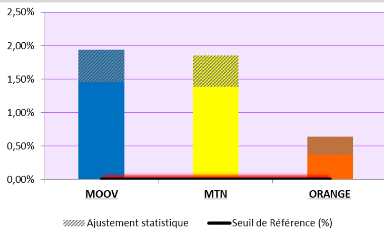
Taux de débit moyen en Uplink par session d'utilisateur inférieur à 512 kb/s (Tddu)
